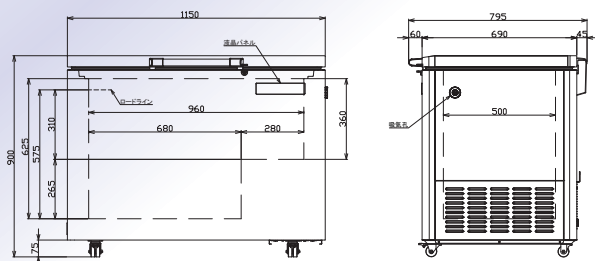
寸法図面
