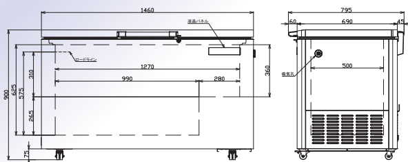
寸法図面
