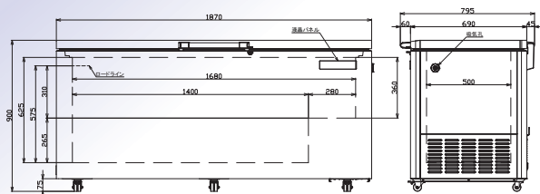
寸法図面
