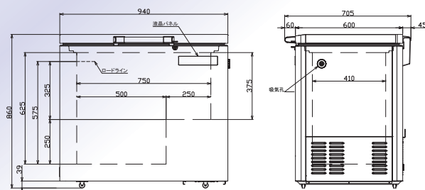
寸法図面
