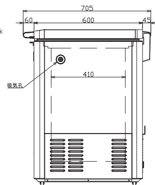
寸法図面
