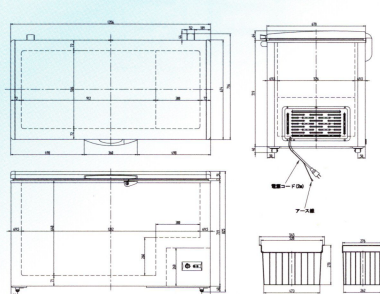
寸法図面
