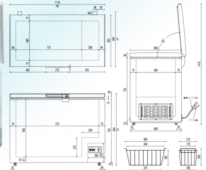
寸法図面
