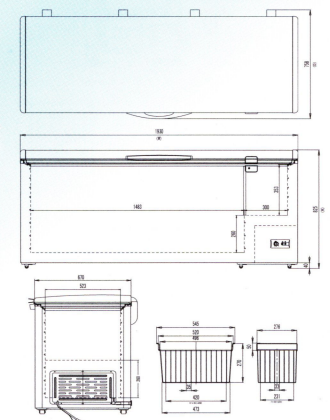
寸法図面
