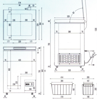
寸法図面
