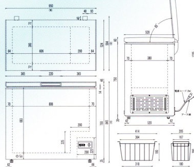
寸法図面
