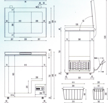
寸法図面
