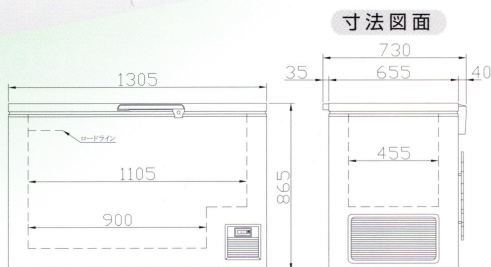
寸法図面
