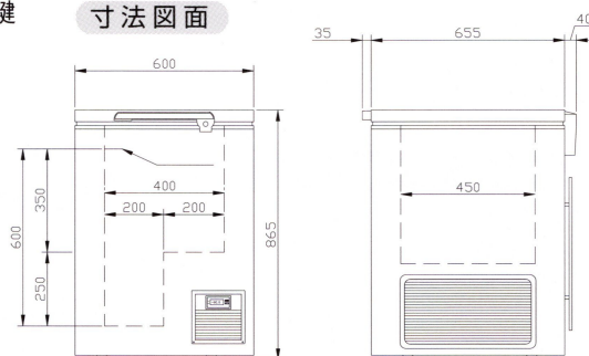
寸法図面
