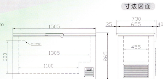
寸法図面
